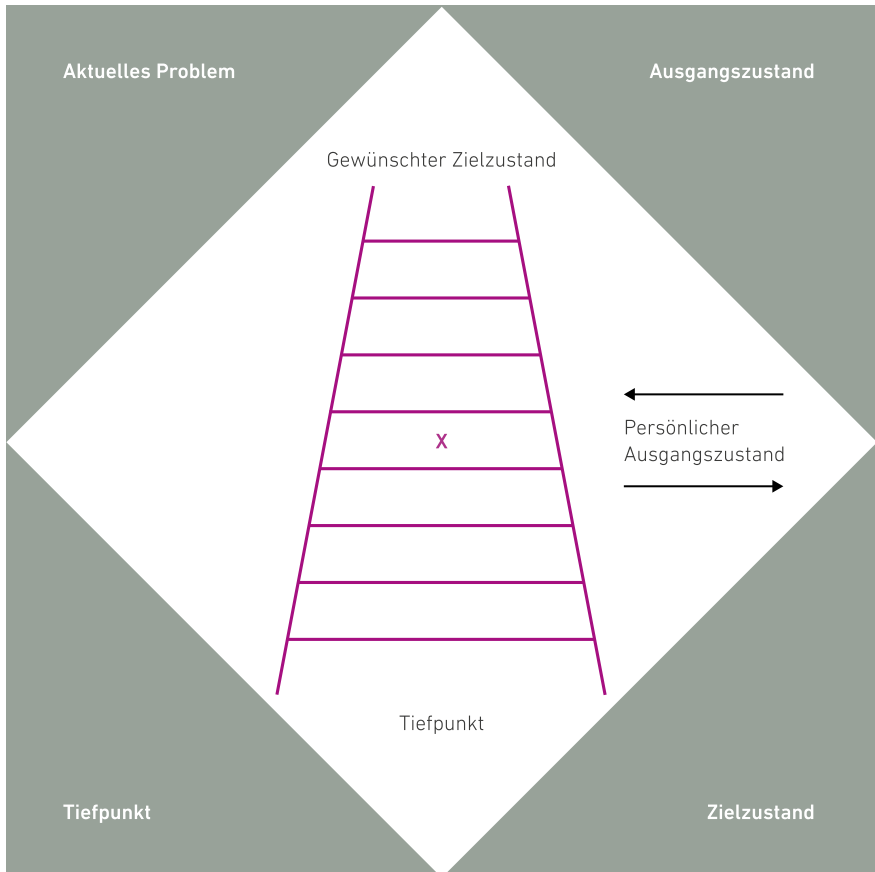
Abbildung 9.3: Entfernung des Standortes zum erwünschten Zielzustand (nach Priestley et al., 1978; Petry, 2003, S. 62)
